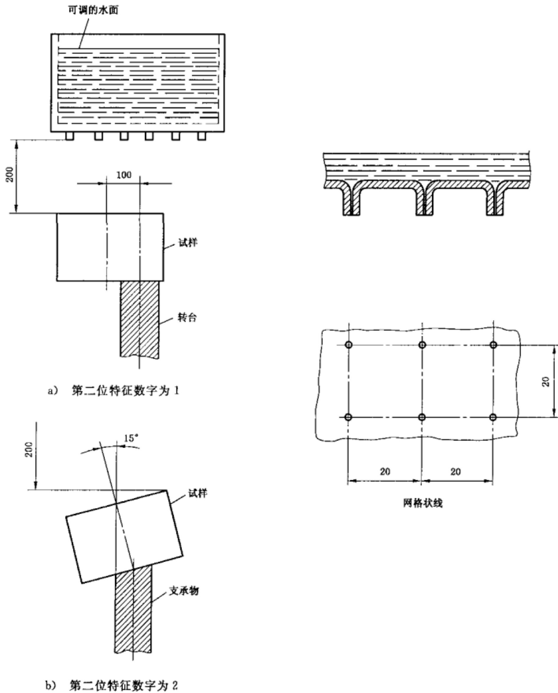
图 3 检验防垂直滴水试验装置(滴水箱)
